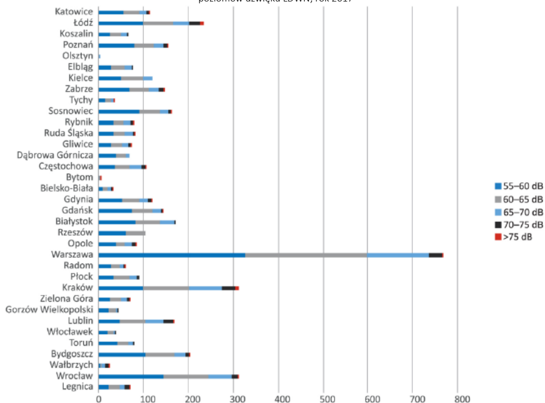
Ryc. 25. Hałas drogowy w aglomeracjach – liczba mieszkańców (w tysiącach) narażonych na hałas drogowy w poszczególnych klasach poziomów dźwięku LDWN; rok 2017
