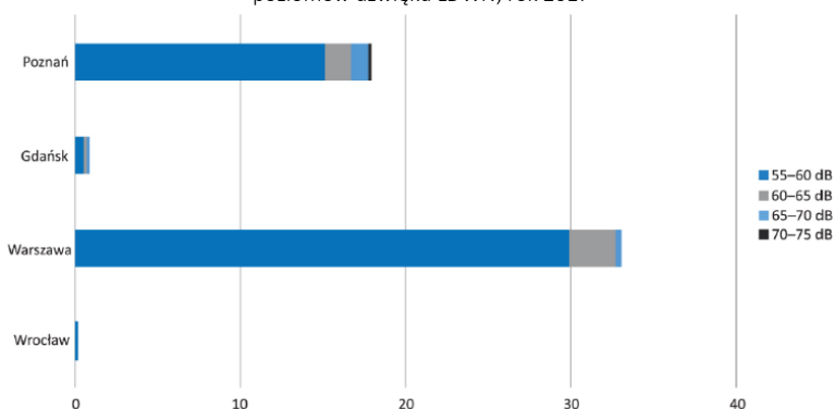
Ryc. 27. Hałas lotniczy w aglomeracjach – liczba mieszkańców (w tysiącach) narażonych na hałas lotniczy w poszczególnych klasach poziomów dźwięku LDWN; rok 2017
