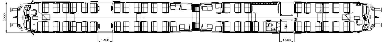
Widok rozplanowania wnętrza wariant 1 (standardowa kabina WC)
