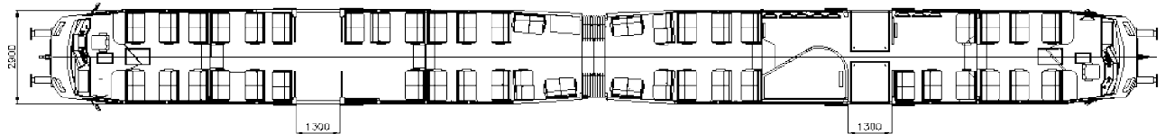
Widok rozplanowania wnętrza wariant 1 (standardowa kabina WC)
