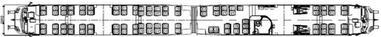
Widok rozplanowania wnętrza wariant 2 (duże kabina WC)
