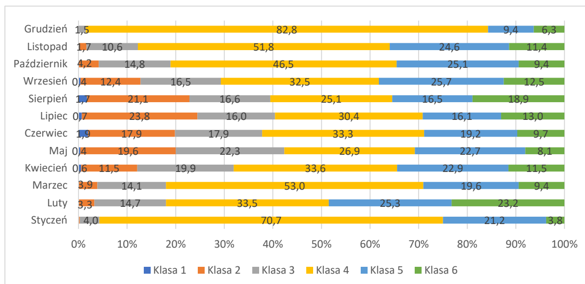
Rysunek 1-13 Udział [%] klas równowagi atmosfery Pasquilla wyznaczonych przez model WRF/CALMET, w strefie miasta Kalisz w poszczególnych miesiącach w 2018 r.
