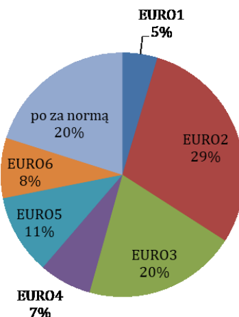
Rysunek 1-70 Flota samochodów osobowych wg. norm EURO w Polsce w 2018 r.
