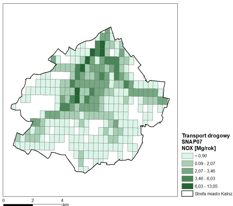
Rysunek 1-52 Rozmieszczenie oraz ładunki emisji liniowej tlenków azotu w transporcie drogowym (SNAP 07) w strefie miasto Kalisz w 2018 r.
