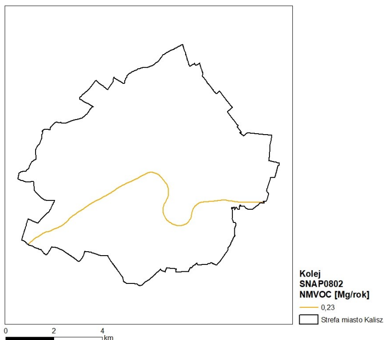
Rysunek 1-58 Rozmieszczenie oraz ładunki emisji liniowej niemetanowych lotnych związków organicznych w transporcie kolejowym (SNAP 0802) w strefie miasto Kalisz w 2018 r.
