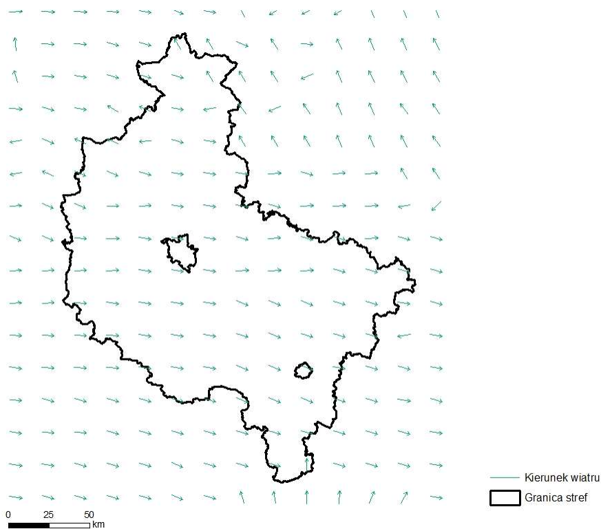
Rysunek 1-6 Dominujący w roku kierunek wiatru wyznaczony przez model WRF/CALMET dla strefy wielkopolskiej 2018 r.
