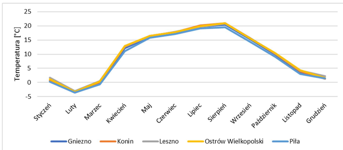
Rysunek 1-15 Przebiegi średnich miesięcznych temperatur powietrza wyznaczone przez model WRF/CALMET w strefie wielkopolskiej w 2018 r.
