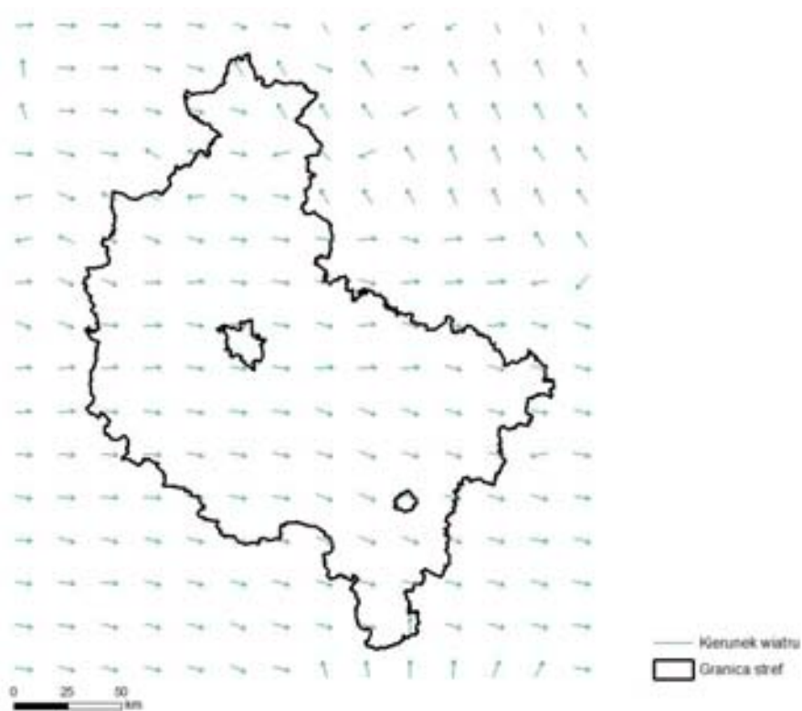
Rysunek 1-6 Dominujący w 2018 roku kierunek wiatru wyznaczony przez model WRF/CALMET dla strefy wielkopolskiej
