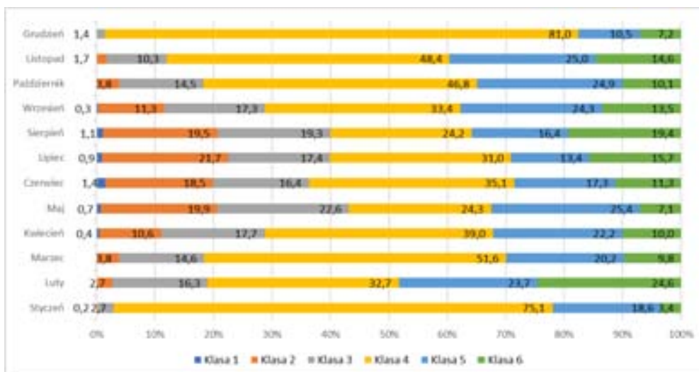
Rysunek 1-16 Udział klas równowagi atmosfery Pasquilla wyznaczonych przez model WRF/CALMET, w strefie wielkopolskiej w poszczególnych miesiącach w 2018 r.
