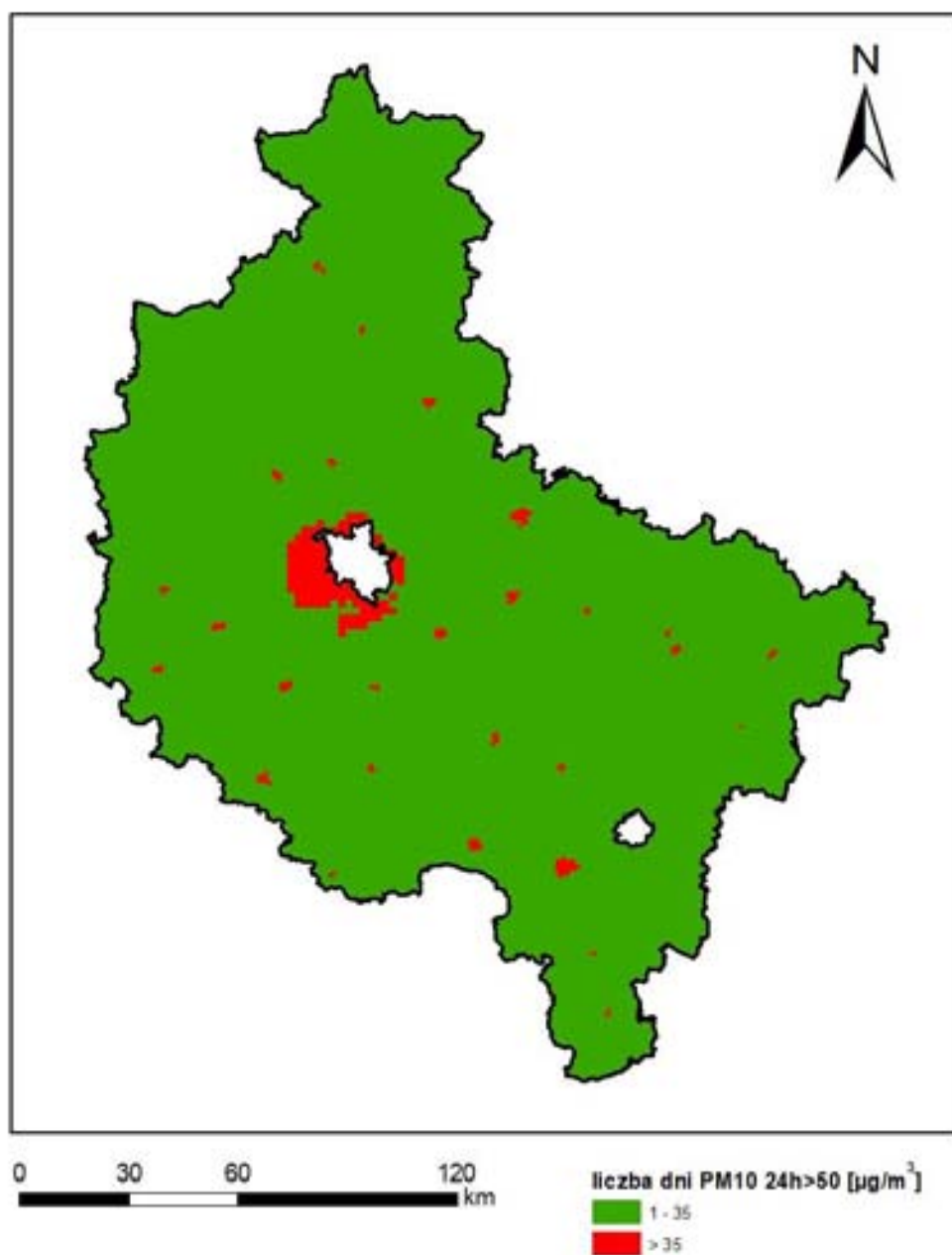
Rysunek 3-3 Liczba dni z przekroczeniami średniego dobrego poziomu dopuszczalnego pyłu zawieszonego PM10 w strefie wielkopolskiej w 2018 roku
