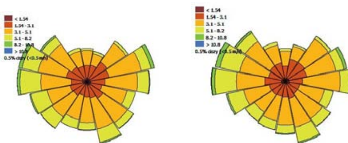
Rysunek 1-10 Częstość % występowania prędkości wiatru w określonych przedziałach w strefie wielkopolskiej w 2018 r.
