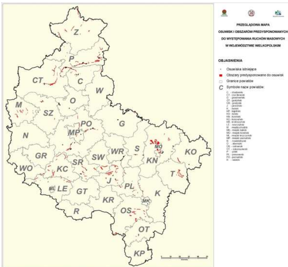
Ryc. 22 Mapa osuwisk i terenów predysponowanych do występowania ruchów masowych na terenie województwa wielkopolskiego (wg PIG-PIB)
