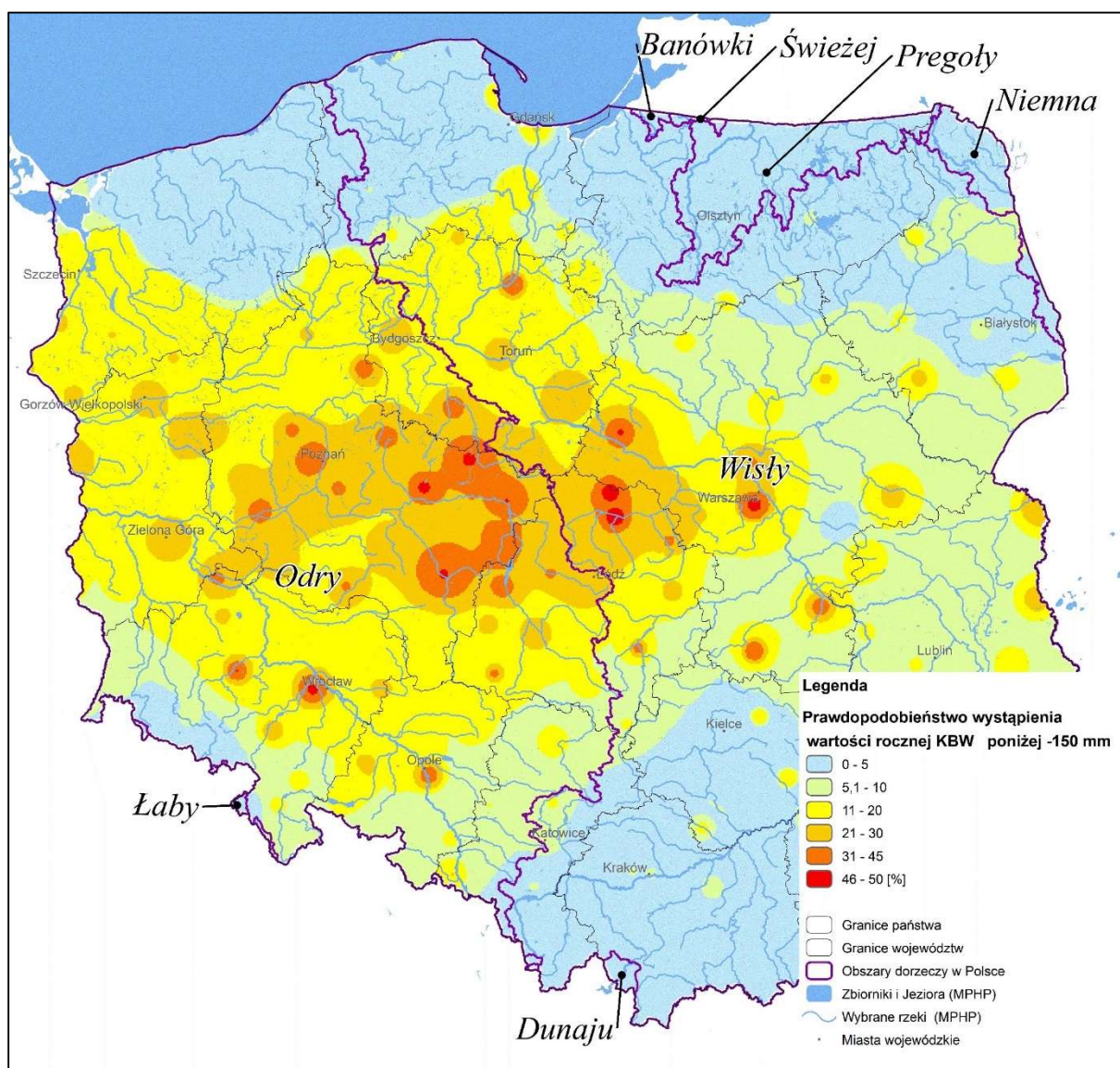
Ryc. 17 Prawdopodobieństwo wystąpienia wartości rocznej KBW poniżej -150 mm (1987 - 2018)
