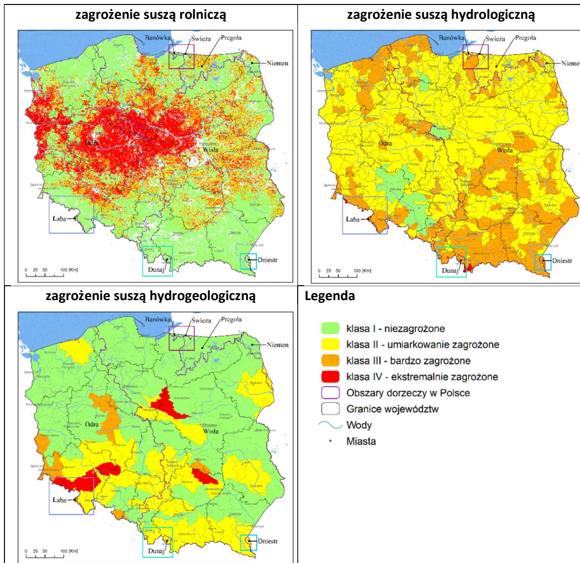
Ryc. 18 Zagrożenie zjawiskiem suszy poszczególnych typów
