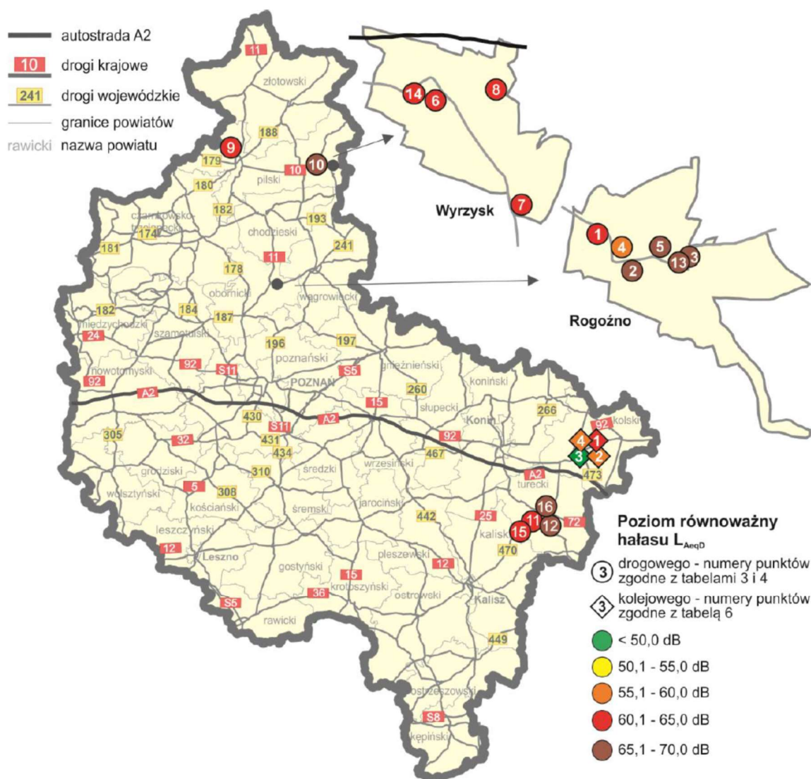
Ryc. 8. Wyniki pomiarów hałasu komunikacyjnego prowadzonych w Wielkopolsce w porze dziennej w 2019 r.
