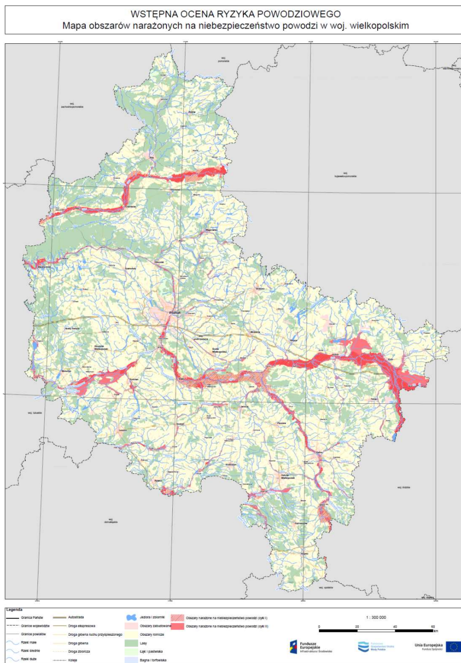
Ryc. 14. Obszary narażone na niebezpieczeństwo powodzi w województwie wielkopolskim
