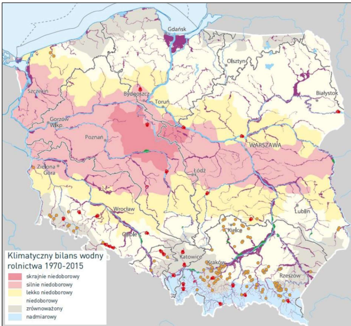
Ryc. 16 Klimatyczny bilans wodny Polski dla wielolecia 1970-2015
