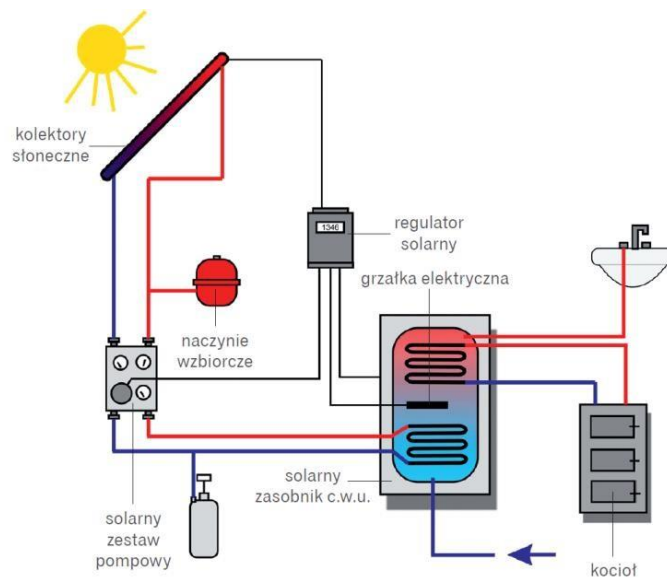
Schemat instalacji kolektorów słonecznych (www.budujemydom.pl)
