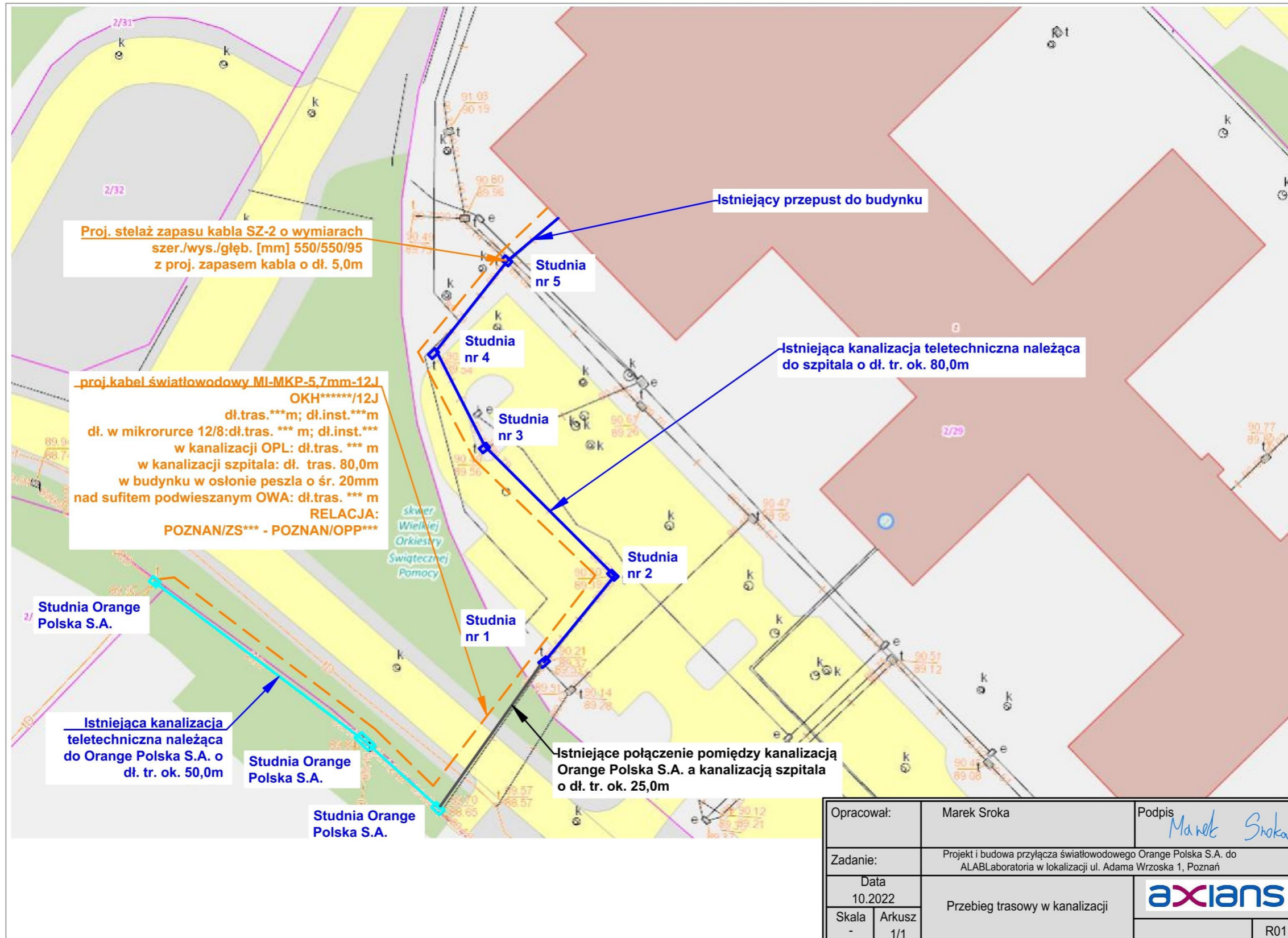
Plan przebiegu trasy projektowanej linii światłowodowej na nieruchomości położonej w Poznaniu, przy ul. A. Wrzoska 1
