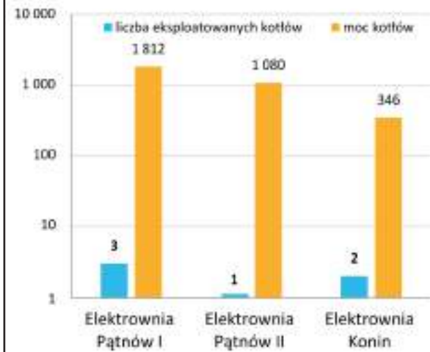
Liczba i moc eksploatowanych kotłów [MW]
