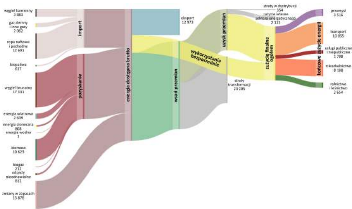
Wykres 11. Bilans energetyczny dla Wielkopolski Wschodniej dla roku 2022 [TJ].
