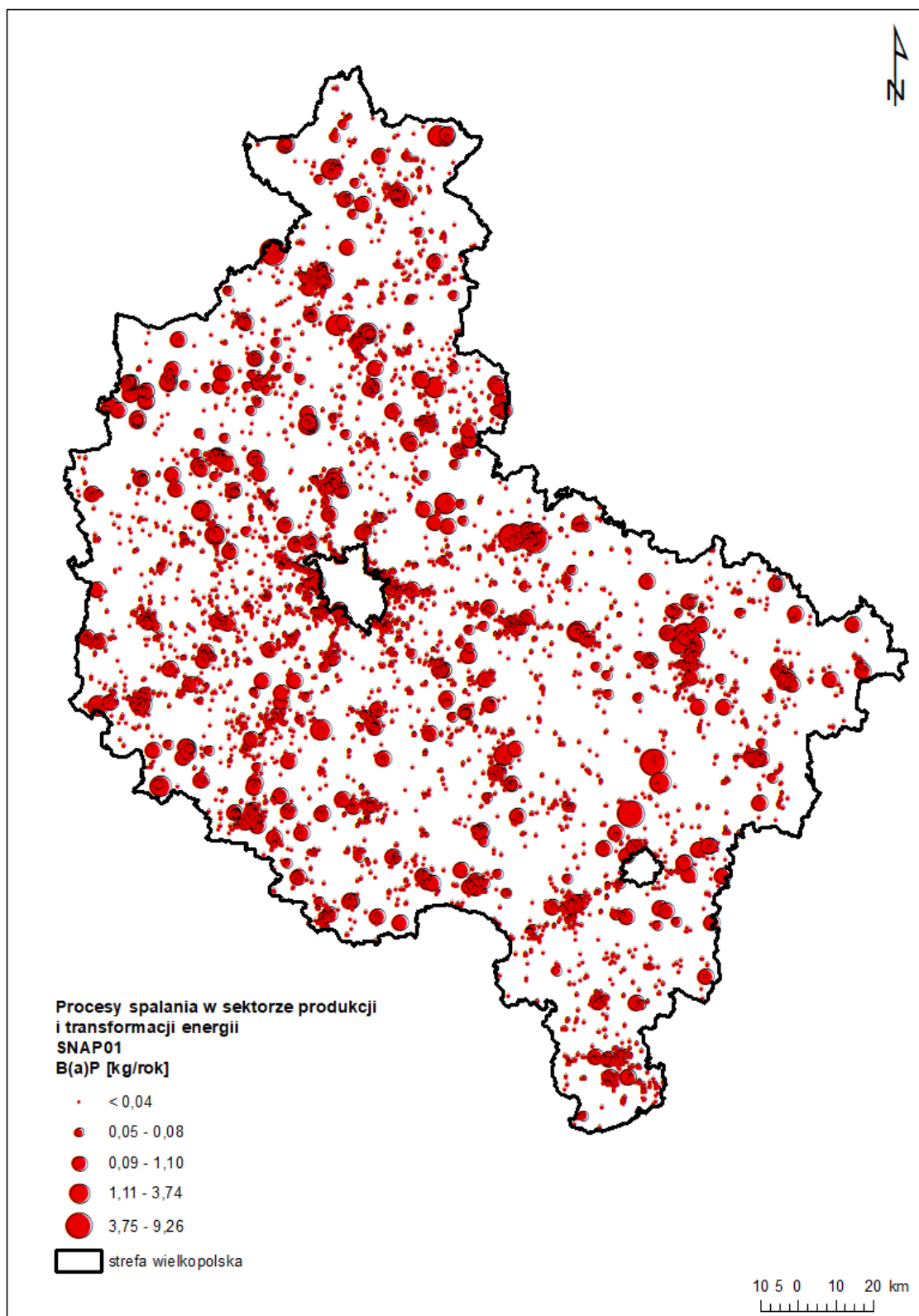
Rysunek 19 Rozmieszczenie oraz ładunki emisji punktowej benzo(a)pirenu [kg/rok] w sektorze produkcji i transformacji energii (SNAP 01) w strefie wielkopolskiej w 2024 r.
