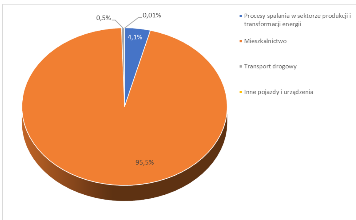
Rysunek 14 Udziały [%] poszczególnych typów emisji z napływu wg kategorii SNAP w łącznej emisji napływowej B(a)P dla strefy wielkopolskiej w 2024 r.
