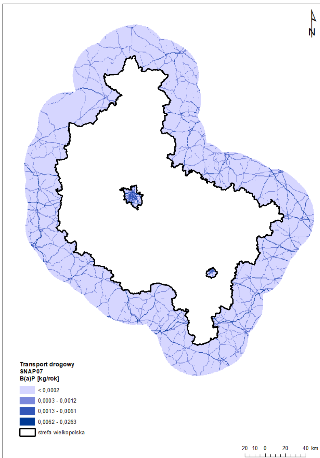
Rysunek 17 Rozmieszczenie oraz ładunki napływowej emisji powierzchniowej benzo(a)pirenu [kg/rok] dla strefy wielkopolskiej w sektorze transportu drogowego (SNAP 07) w 2024 r.
