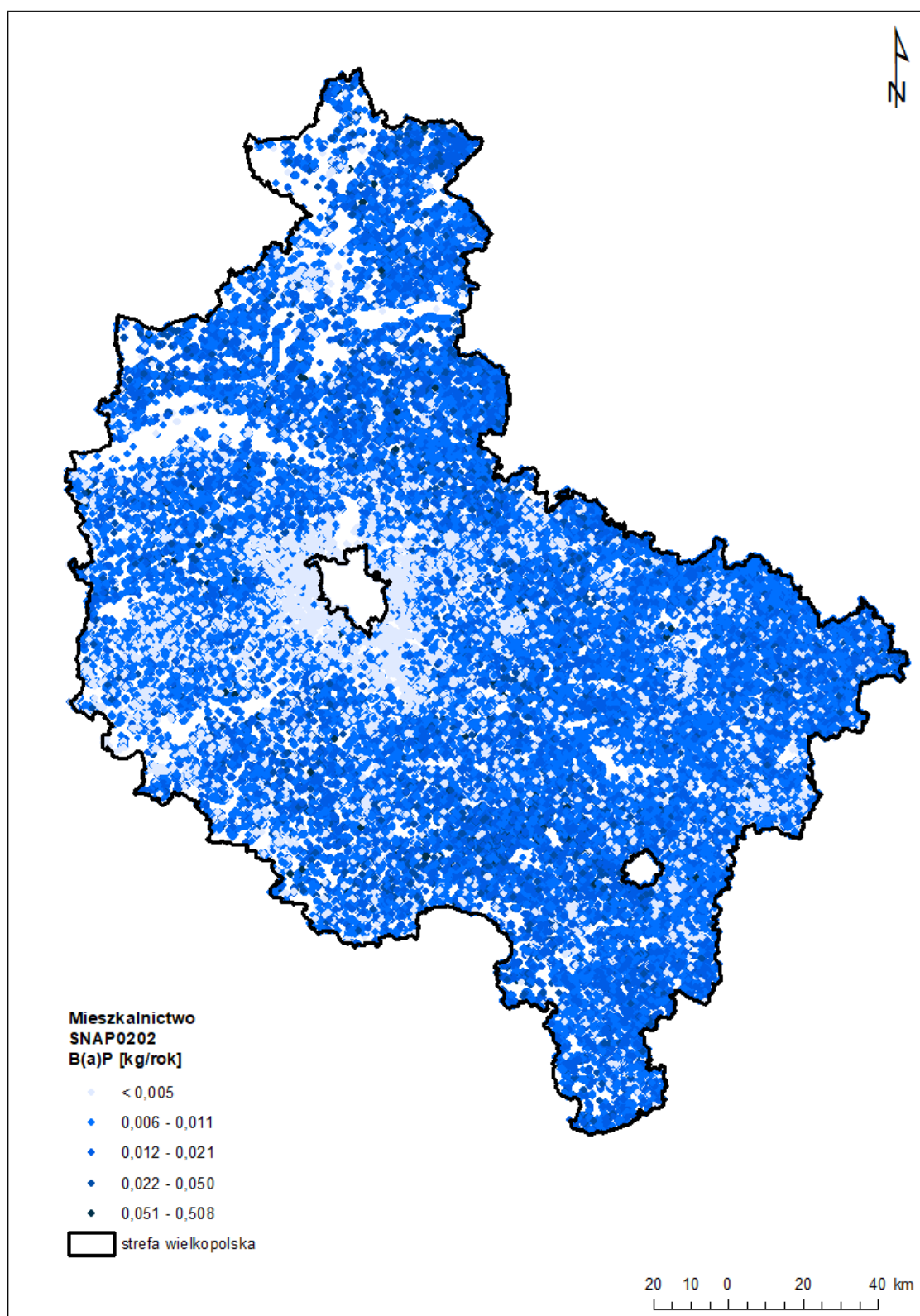
Rysunek 20 Rozmieszczenie oraz ładunki emisji powierzchniowej benzo(a)pirenu [kg/rok] w sektorze mieszkalnictwa (SNAP 0202) w strefie wielkopolskiej w 2024 r.
