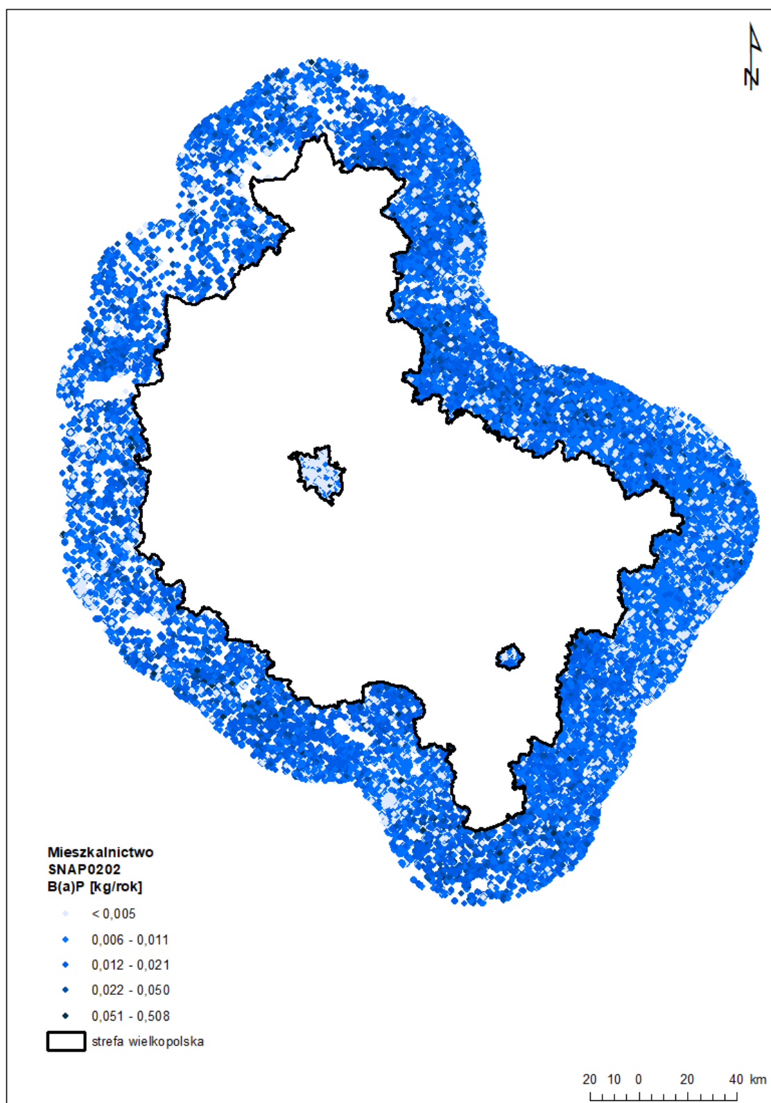
Rysunek 16 Rozmieszczenie oraz ładunki napływowej emisji powierzchniowej benzo(a)pirenu [kg/rok] dla strefy wielkopolskiej w sektorze mieszkalnictwa (SNAP 0202) w 2024 r.
