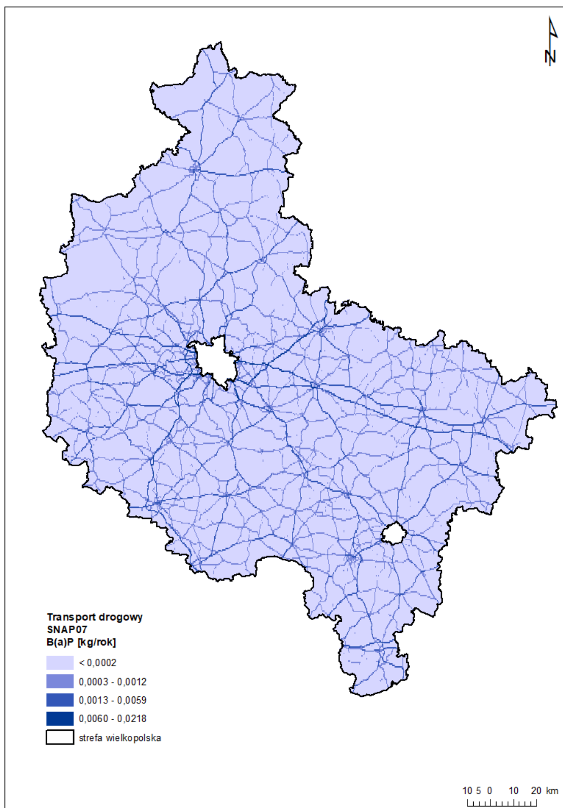
Rysunek 21 Rozmieszczenie oraz ładunki emisji powierzchniowej benzo(a)pirenu [kg/rok] w sektorze transportu drogowego (SNAP 07) w strefie wielkopolskiej w 2024 r.
