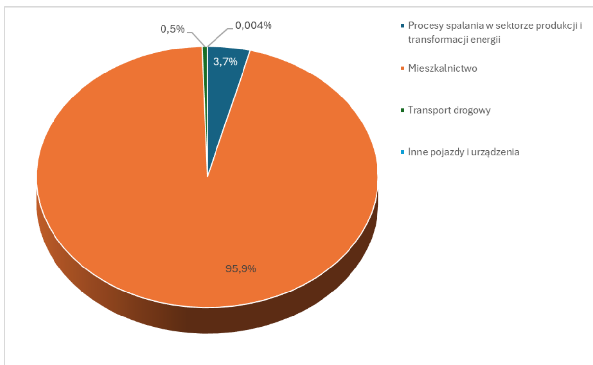
Rysunek 18 Udziały [%] poszczególnych typów emisji, wg kategorii SNAP w emisji B(a)P w strefie wielkopolskiej w 2024 r.
