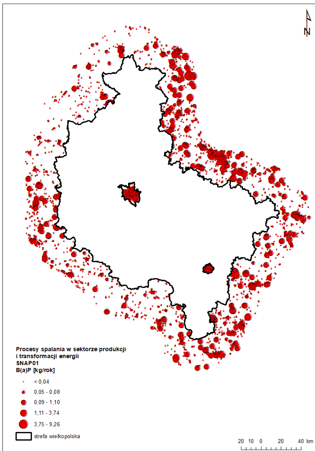
Rysunek 15 Rozmieszczenie oraz ładunki napływowej emisji punktowej benzo(a)pirenu [kg/rok] dla strefy wielkopolskiej w sektorze produkcji i transformacji energii (SNAP 01) w 2024 r.
