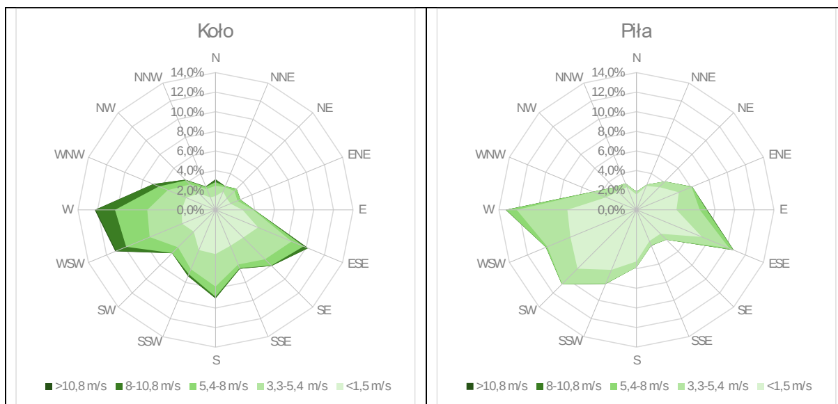
Rysunek 6 Różnice wiatru dla stacji pomiarowych w Lesznie, Kole i w Pile w strefie wielkopolskiej dla 2024 r.
