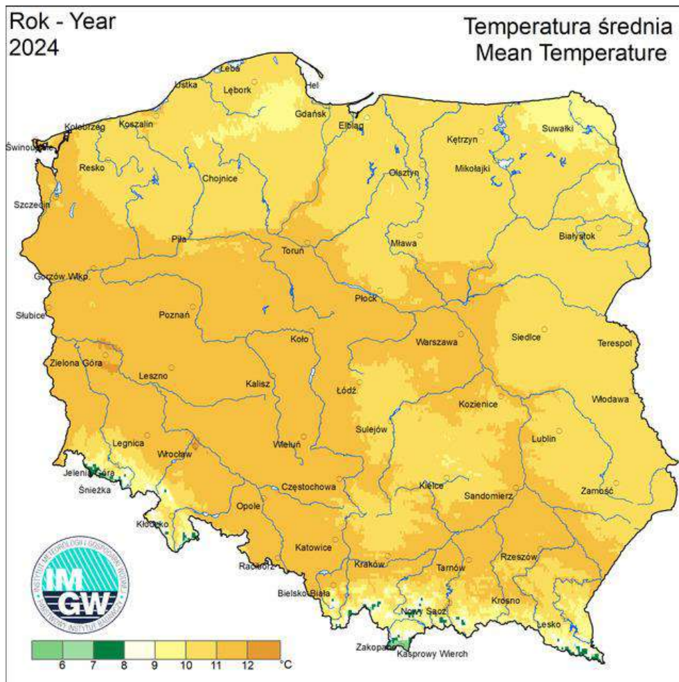
Rysunek 7 Przestrzenny rozkład średniej rocznej temperatury powietrza [°C] w Polsce w 2024 roku
