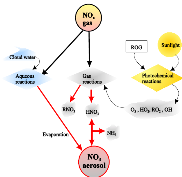
Rysunek 43 Procesy utleniania tlenków azotu w atmosferze wykorzystane w mechanizmie MESOPUFF II w modelu CALPUFF
