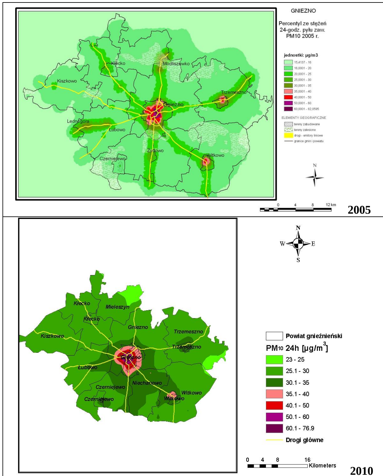
Rysunek 68 Zestawienie wyników modelowania stężeń pyłu zawieszonego PM 10 o okresie uśredniania wyników pomiarów 24 godziny pochodzących z emisji łącznej z terenu powiatu gnieźnieńskiego w latach 2005 i 2010
