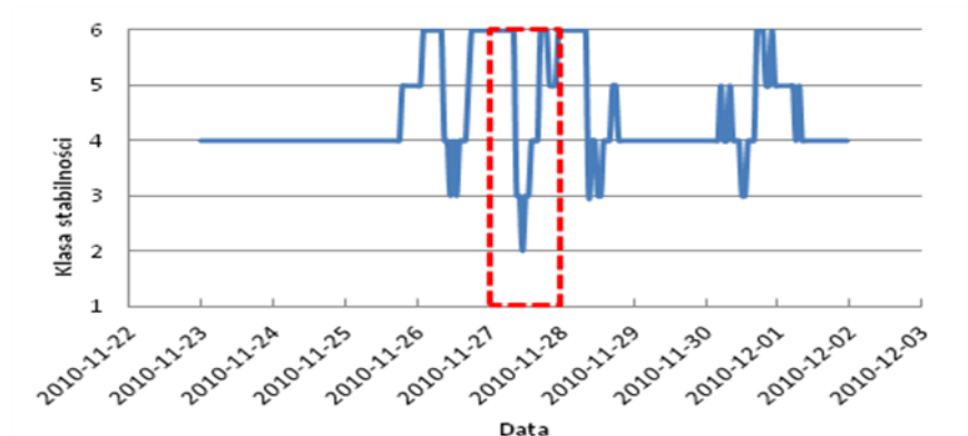
Rysunek 6 Klasy równowagi atmosfery w Gnieźnie 27 listopada 2010 r.
