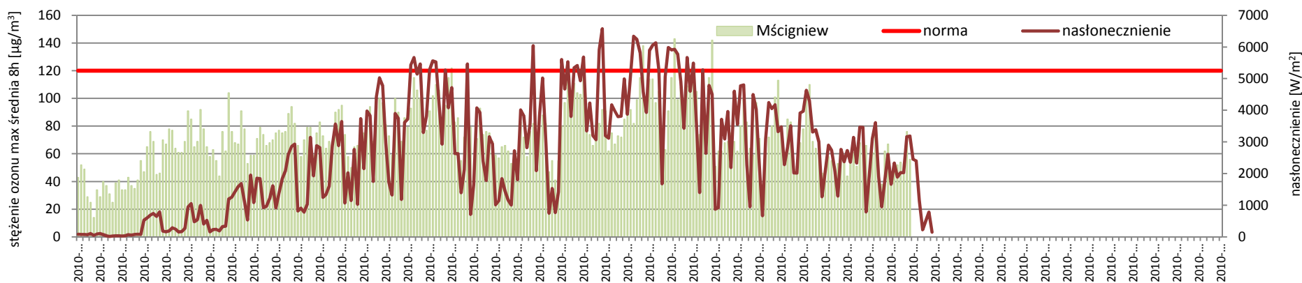
Rysunek 9. Przebieg zmienności maksymalnych dobowych kroczących średnich ośmiogodzinnych stężeń ozonu w 2009 roku w Mścigniewie w zestawieniu z nasłonecznieniem 35
