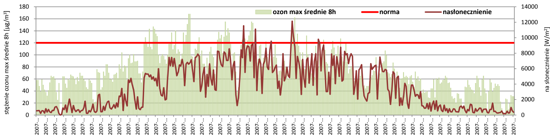
Rysunek 3. Przebieg zmienności maksymalnych dobowych kroczących średnich ośmiogodzinnych stężeń ozonu w 2007 roku w Krzyżówce w zestawieniu z nasłonecznieniem 29
