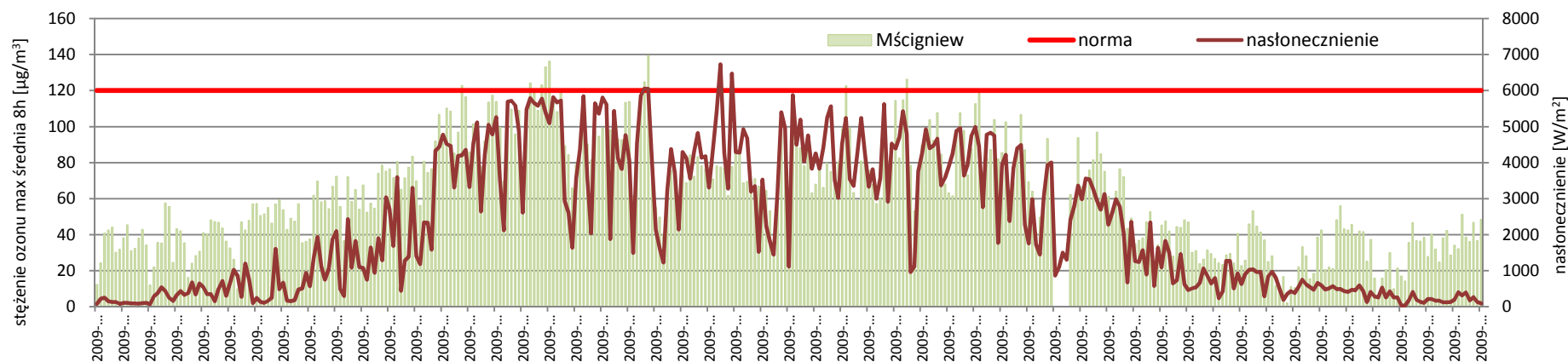
Rysunek 9. Przebieg zmienności maksymalnych dobowych kroczących średnich ośmiogodzinnych stężeń ozonu w 2009 roku w Mścigniewie w zestawieniu z nasłonecznieniem 35
