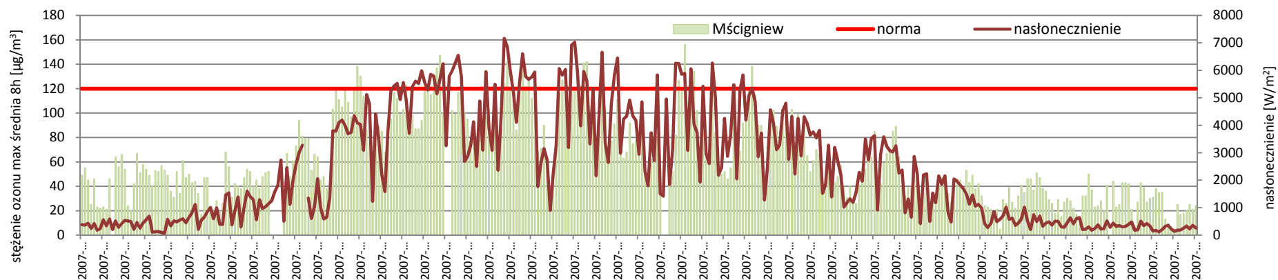
Rysunek 7. Przebieg zmienności maksymalnych dobowych kroczących średnich ośmiogodzinnych stężeń ozonu w 2007 roku w Mścigniewie w zestawieniu z nasłonecznieniem 33
