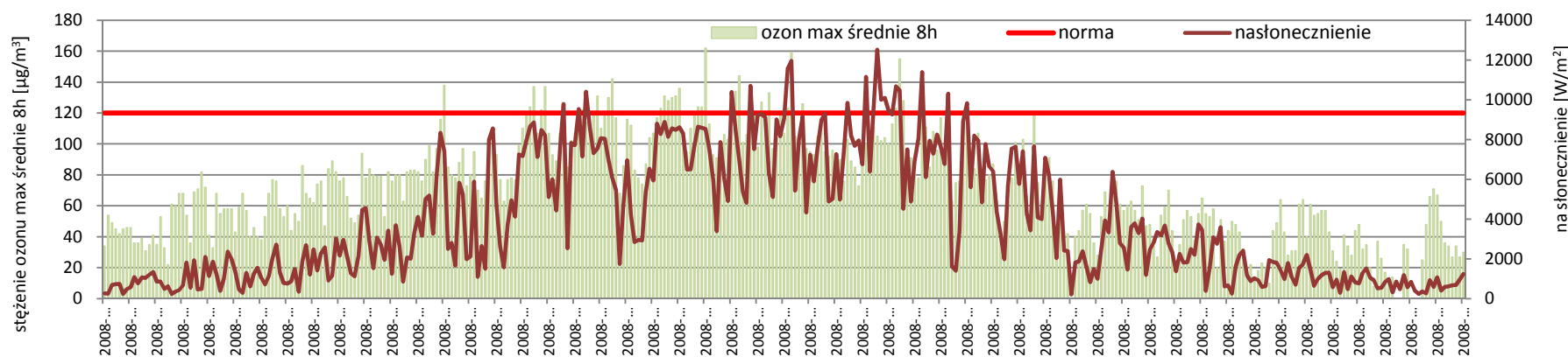
Rysunek 4. Przebieg zmienności maksymalnych dobowych kroczących średnich ośmiogodzinnych stężeń ozonu w 2008 roku w Krzyżówce w zestawieniu z nasłonecznieniem 30
